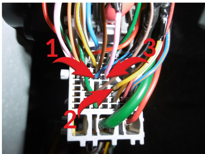
Подключение к цепям запуска двигателя 1 - Зажигание 1 (синий/черный провод); 2 - Зажигание 2 (желтый провод); 3 - Стартер (розовый провод).
