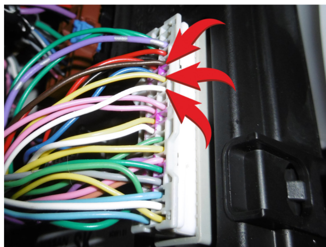
Подключение зажигания:
