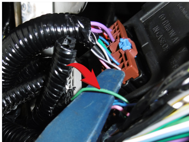
Подключение стартера: зеленый провод, контакт № 19
