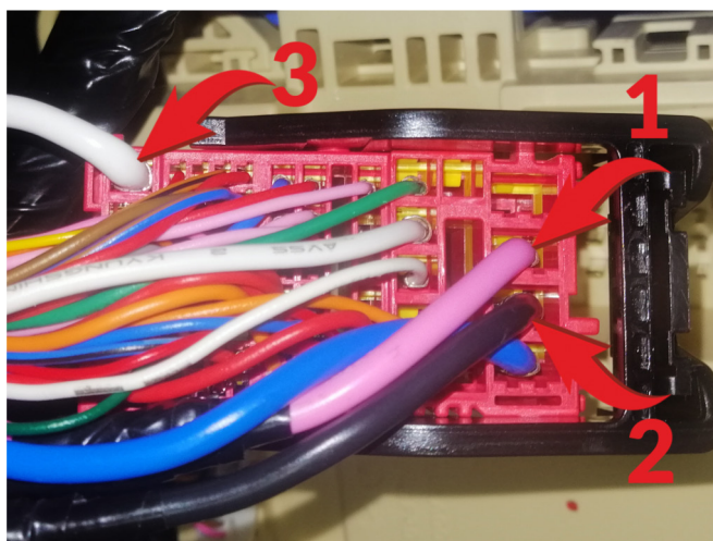
Подключение к цепям запуска двигателя 1 - Зажигание 1 (розовый провод, контакт №21); 2 - Зажигание 2 (черный провод, контакт №38); 3 - Стартер (белый провод, контакт №58).
