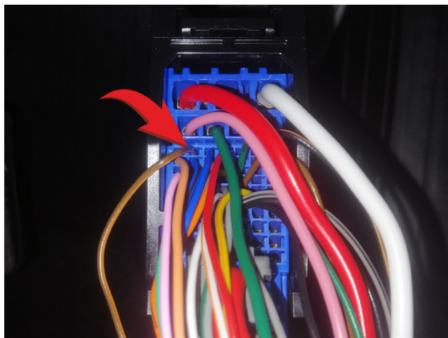
Шина данных (коричневый/оранжевый провод, контакт №23)
