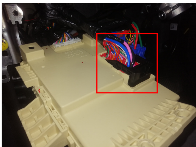
Место подключения цепей запуска двигателя
