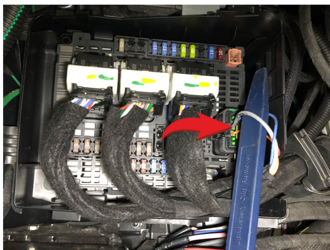
Подключение стартера (серый провод, контакт № 4)
