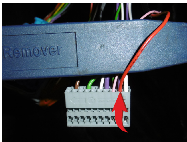
Подключение зажигания (красный провод, контакт № 32)
