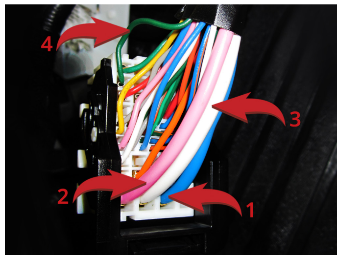
Рис.5 Подключение к силовым цепям запуска двигателя.
