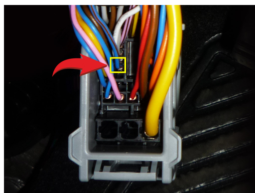
Рис.3 Шина данных (синий/оранжевый провод)
