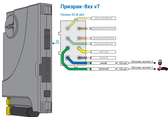
Рис.7 Призрак 8xx подключение ЦЗ
