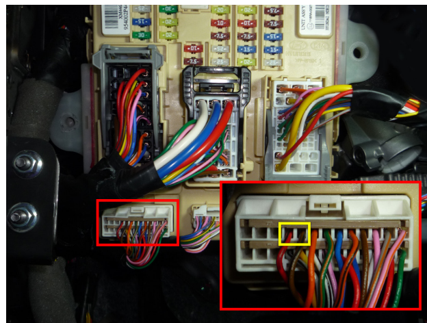
Рис.8 Подключение ЦЗ 1 – Красный/черный - закрытие 2 – Коричневый/черный – открытие
