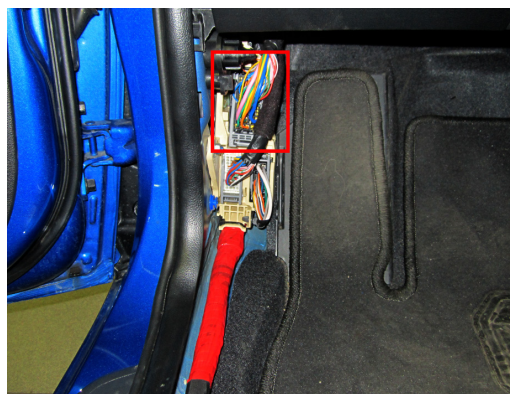
Рис.2 Место подключения
