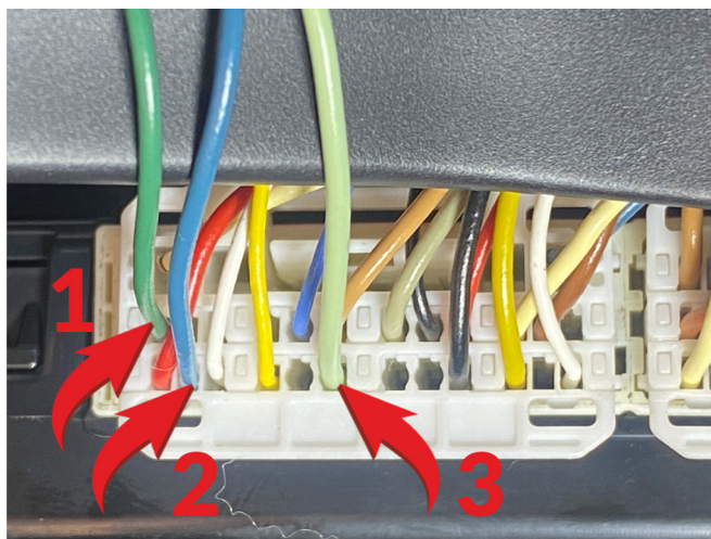
Подключение к цепям автозапуска: 1 - АСС (зеленый провод); 2 - Зажигание 1 (синий провод); 3 - Стартер (салатовый провод).
