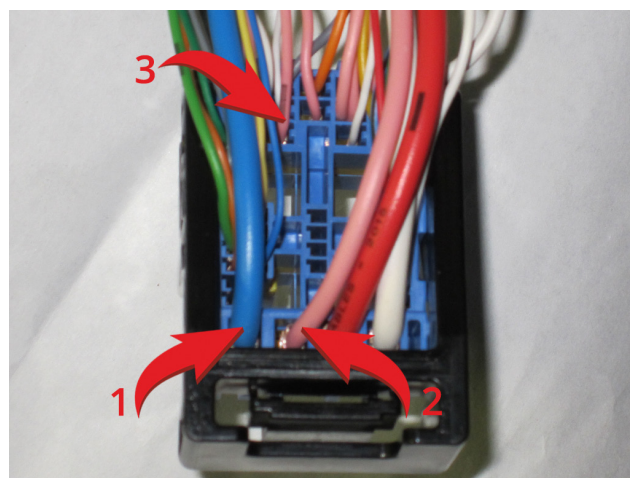
Рис.5 Подключение к силовым цепям запуска двигателя 1 – Зажигание 1 (синий); 2 – Зажигание 2 (розовый); 3 – Стартер (розовый).
