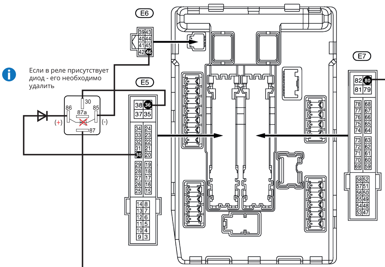
Рис.5 Блок IPDM
