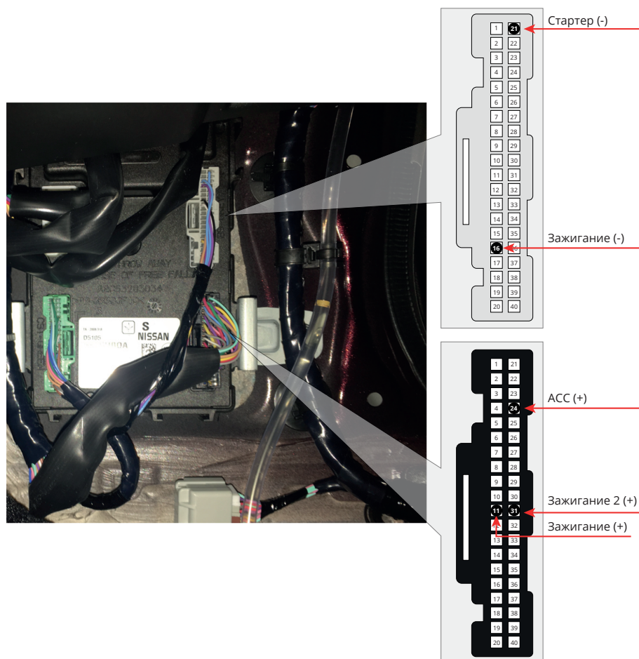
Рис.3 Место подключения к цепям запуска двигателя
