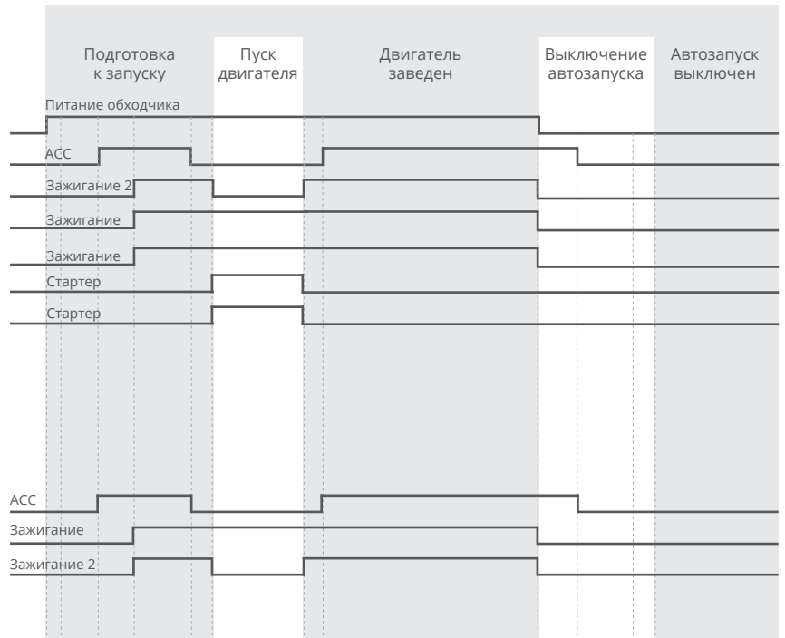
Временная диаграмма работы
