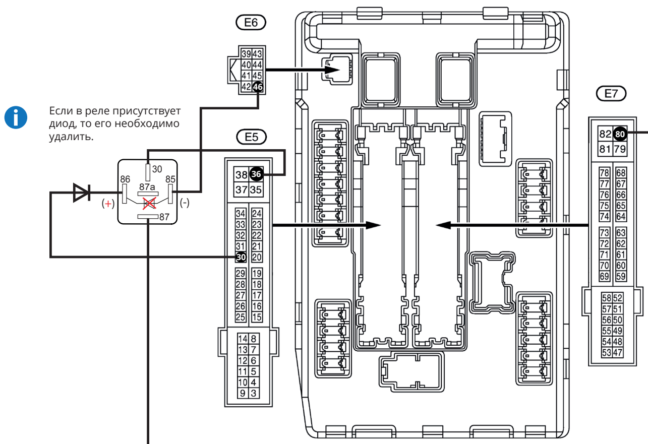
Рис.5 Блок IPDM
