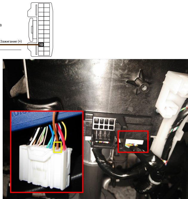
Рис.3 Подключение зажигания
