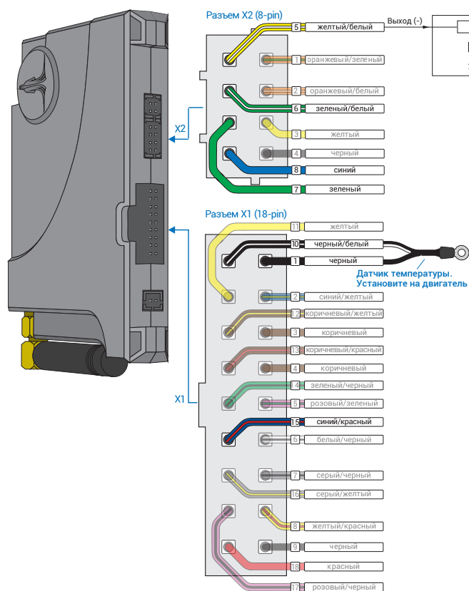
Рис.2 Выходы Призрак-8xx
