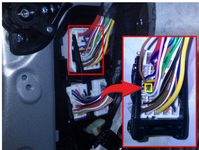
Подключение к шине данных (коричневый/оранжевый провод, контакт №12)
