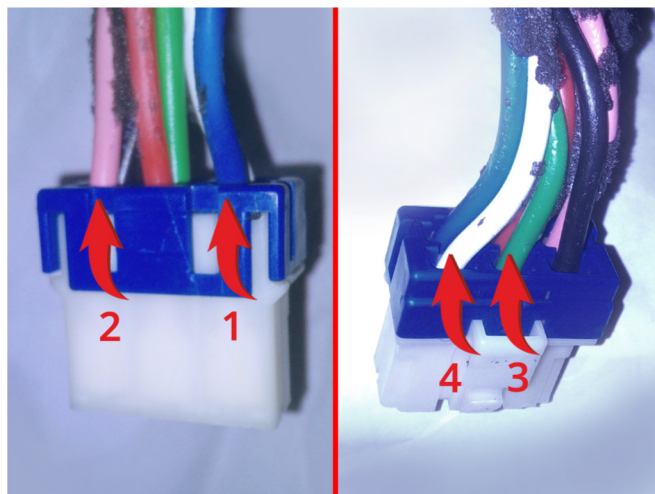
Подключение к силовым цепям запуска двигателя 1 – АСС (синий провод); 2 – Зажигание 1 (розовый провод); 3 – Зажигание 2 (зеленый провод); 4 – Стартер (белый провод).
