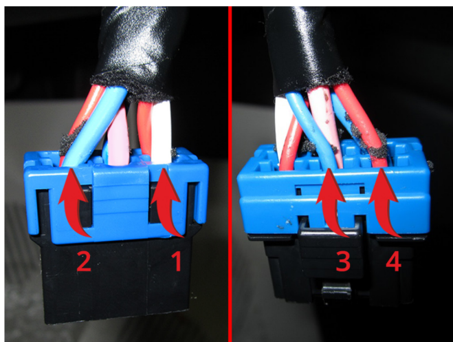
Подключение к силовым цепям запуска двигателя 1 - АКБ (белый провод); 2 - Зажигание 1 (синий провод); 3 - Зажигание 2 (синий провод); 4 - Стартер (красный провод).
