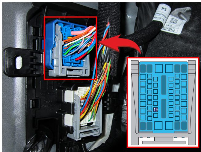
Место подключения (синий/черный провод, контакт №19)
