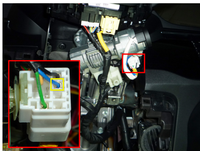
Ключ в замке (синий провод)
