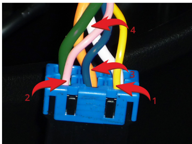
Место подключения у замка зажигания 1 - АСС (желтый провод); 2 - Зажигание 1 (розовый провод); 3 - Зажигание 2 (оранжевый провод); 4 - Стартер (белый провод).
