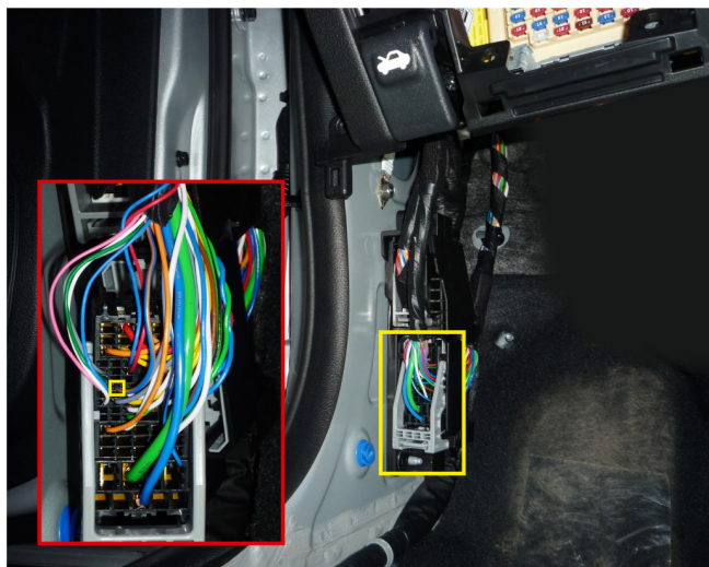
Шина данных (синий/оранжевый провод)
