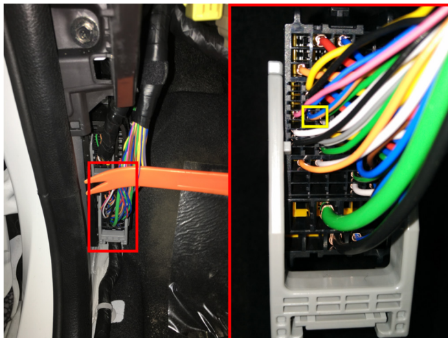
Место подключения к шине данных (синий/оранжевый провод, контакт № 21)
