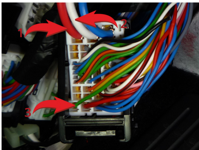
Подключение силовых цепей запуска двигателя 1 – Зажигание 1 (красный провод); 2 – Зажигание 2 (белый провод); 3 – Стартер (зеленый провод).
