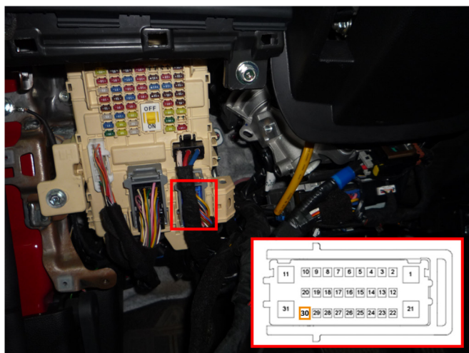
Подключение к силовым цепям запуска двигателя – Стартер (оранжевый провод, контакт №30)
