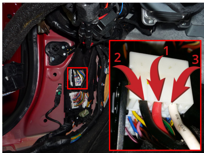
Подключение к силовым цепям запуска двигателя 1 – АСС (красный провод); 2 – Зажигание 1 (черный провод); 3 – Зажигание 2 (белый провод).
