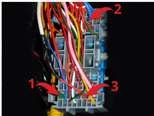
Подключение к силовым цепям запуска двигателя 1 - Зажигание 1 (зеленый провод); 2 - Зажигание 2 (синий провод); 3 - Стартер (красный провод).
