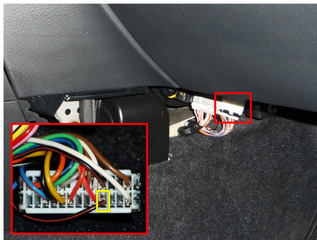
Место подключения (черный/оранжевый провод)
