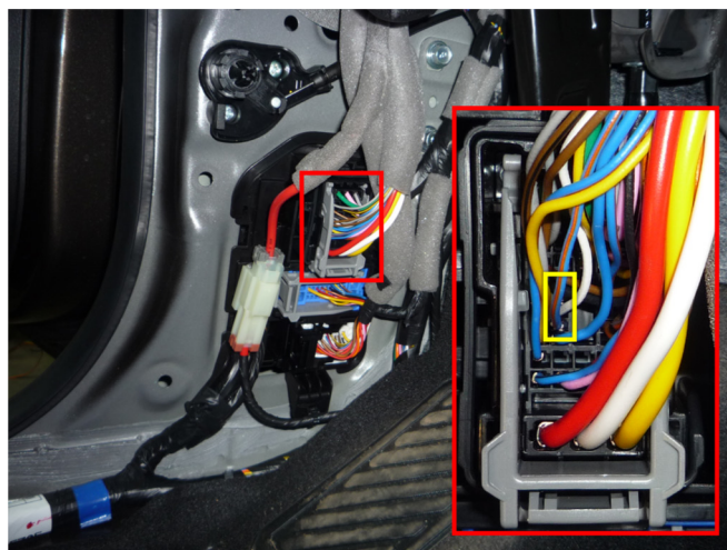
Место подключения (синий/оранжевый провод, контакт №15)
