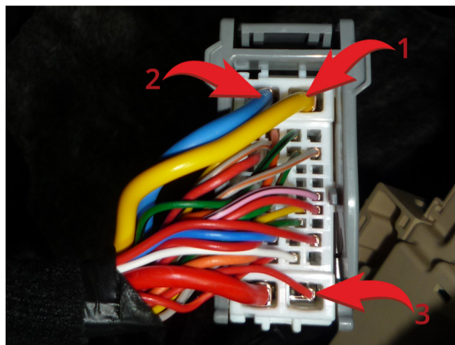
Подключение к цепям запуска двигателя: 1 – Зажигание 1 (желтый провод); 2 – Зажигание 2 (синий провод); 3 – Стартер (красный провод).
