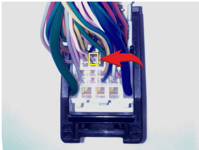
Шина данных (белый/оранжевый провод, контакт №32)
