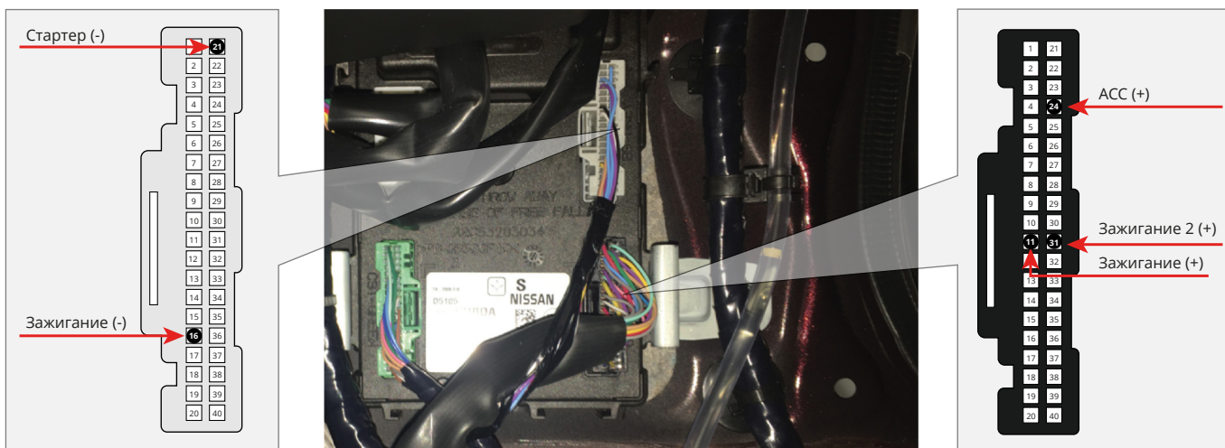
Место подключения к цепям запуска двигателя
