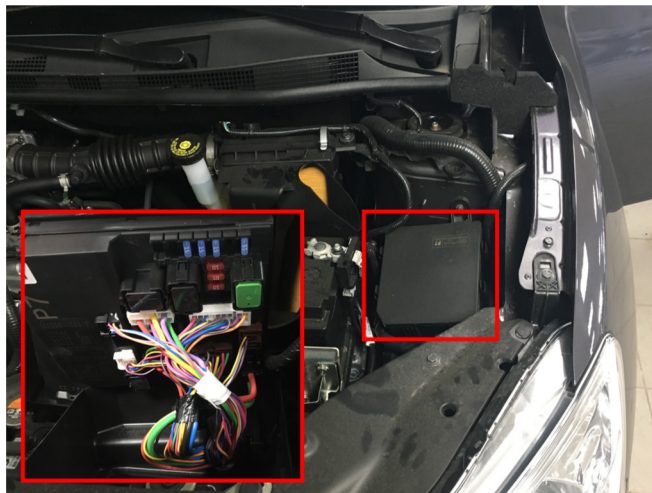
Место подключения реле в блоке IPDMI
