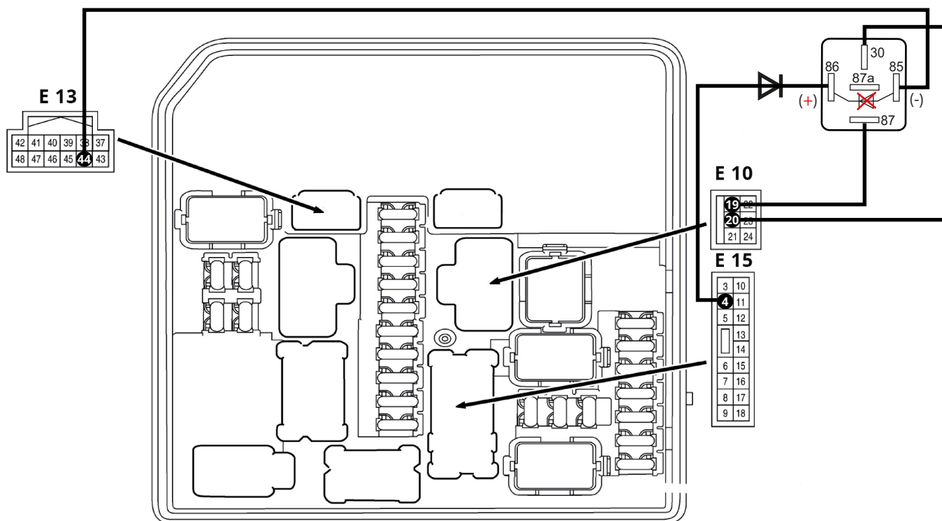
Блок IPDMI
