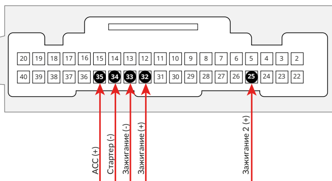
Подключение к цепям запуска двигателя
