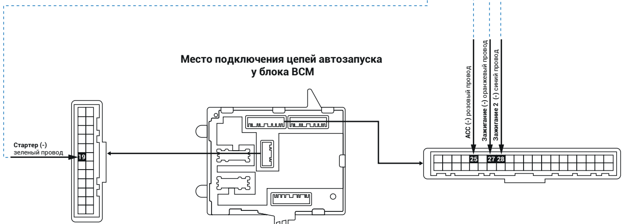
Рис.4 Схема подключения автозапуска
