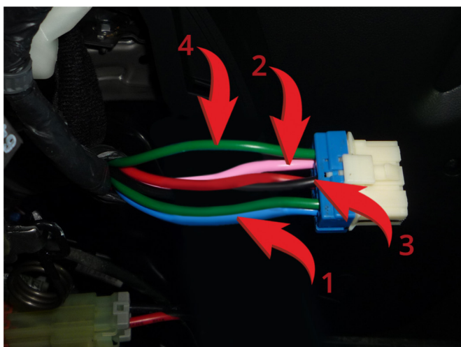
Место подключение к силовым цепям запуска двигателя 1 - АСС (синий провод); 2 - Зажигание 1 (розовый провод); 3 - Зажигание 2 (черный провод); 4 - Стартер (зеленый провод).
