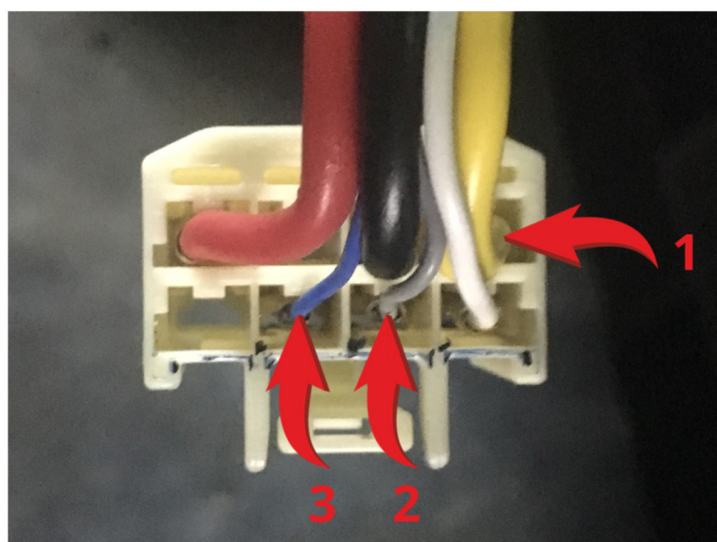
Подключение к цепям замка зажигания 1 – Зажигание (желтый провод); 2 – Зажигание (серый провод); 3 – Стартер (синий провод).
