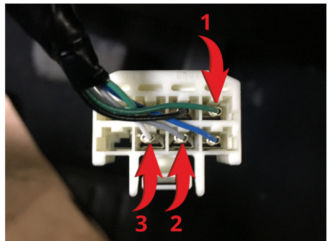
Рис.6 Подключение к цепям замка зажигания
