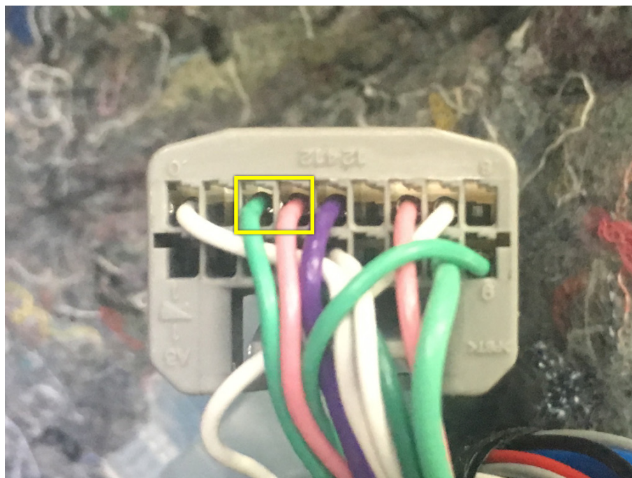
Рис.3 Подключение IMO, IMI
