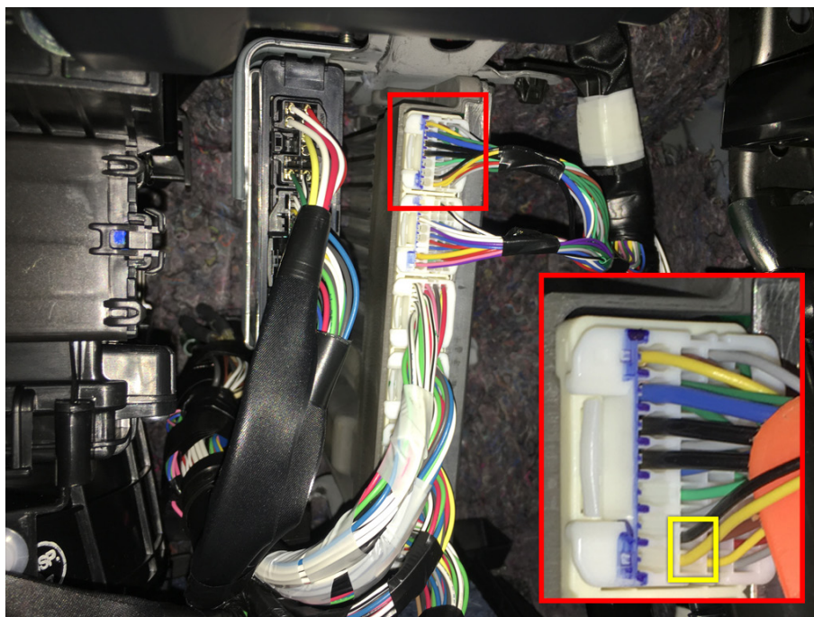
Рис.3 Подключение ИМО, ИМІ (дизель)
