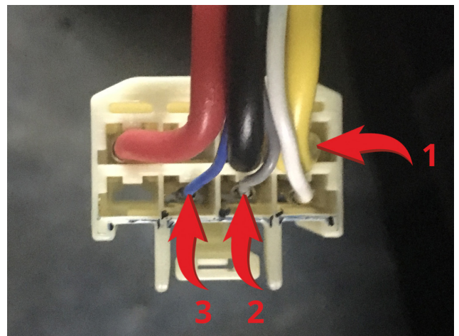
Рис.7 Подключение к цепям замка зажигания.
