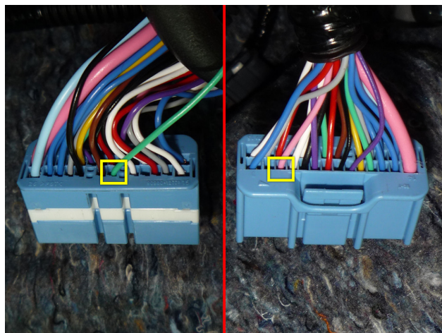
Рис.5 Подключение ИМО, ИМИ
