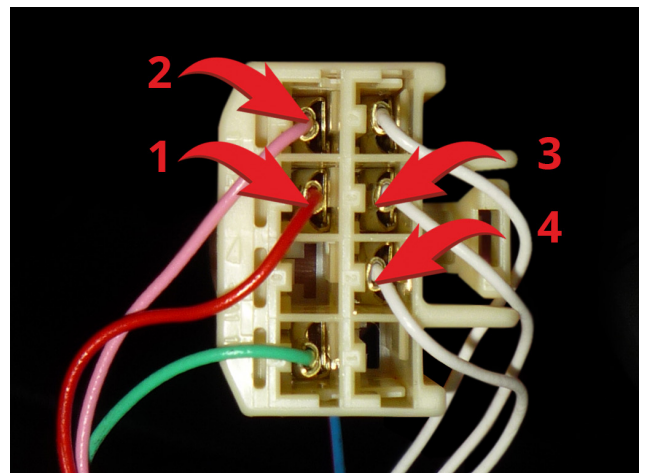
Рис.8 Подключение к цепям замка зажигания.
