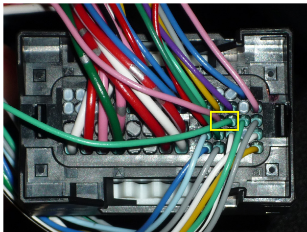
Рис.3 Подключение ИМО, ИМИ
