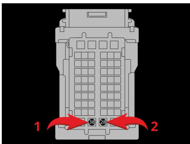
Подключение силовых цепей запуска двигателя 1 - Зажигание 1 (синий провод, контакт №38); 2 - АСС (желтый провод, контакт №28).
