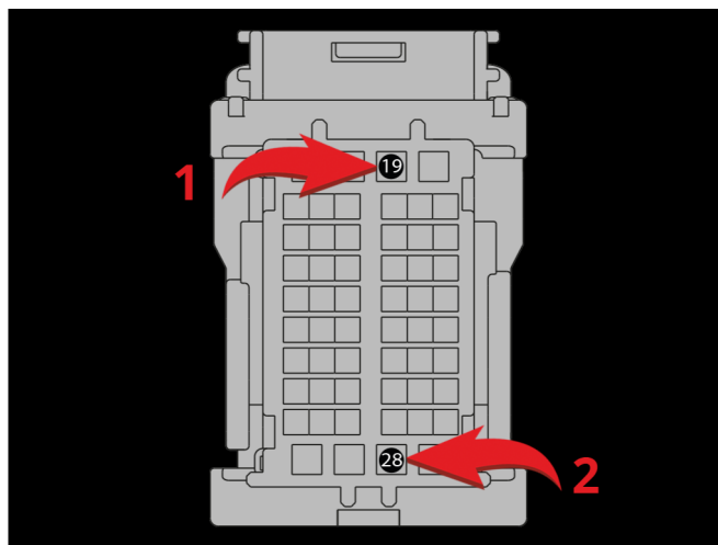
Подключение силовых цепей запуска двигателя 1 - Стартер (розовый провод, контакт №19); 2 - Зажигание 2 (красный провод, контакт №28).
