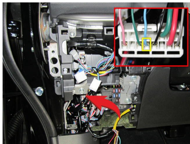
Подключение Стартера (голубой провод)
