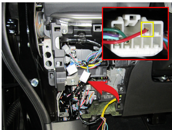
Подключение Зажигания (красный провод)
