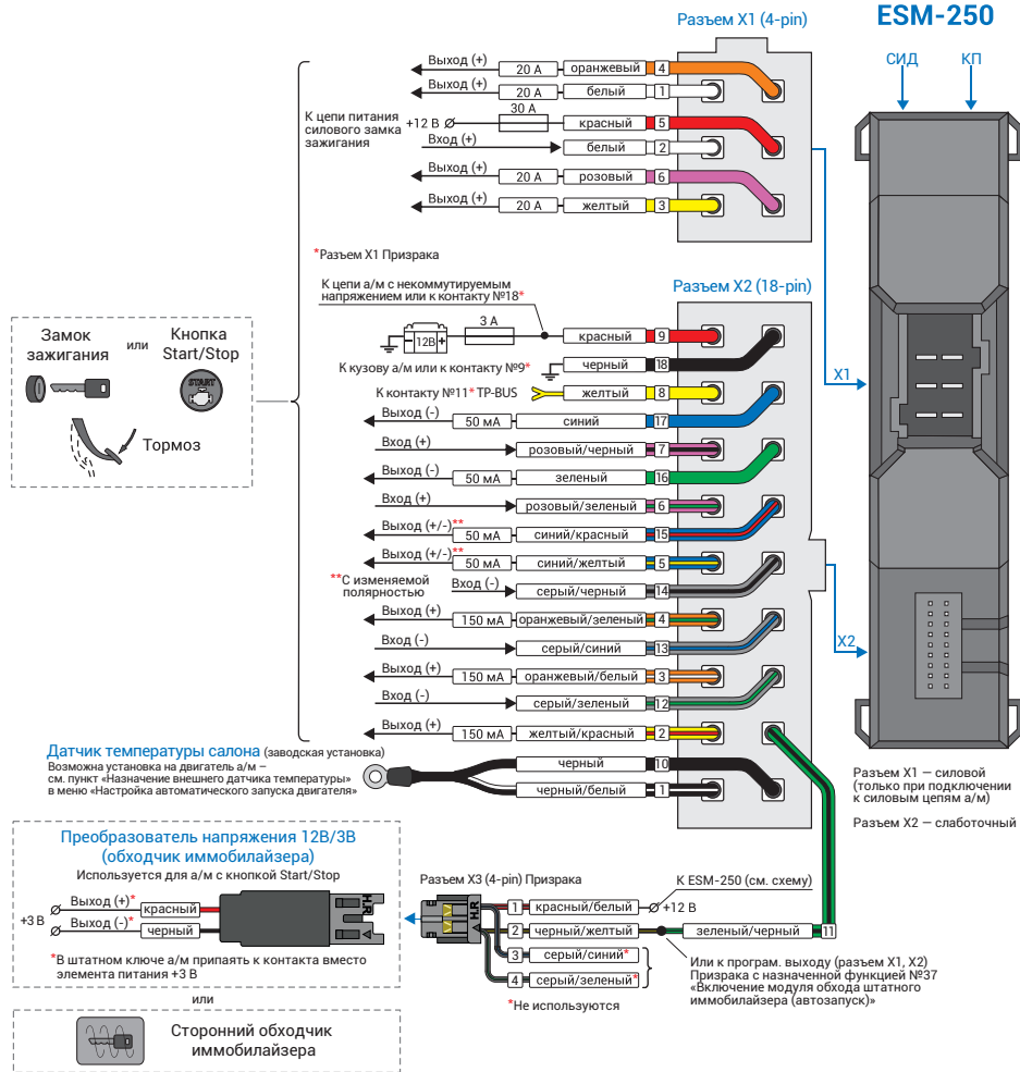
Рис. 2. Назначение выводов модуля
