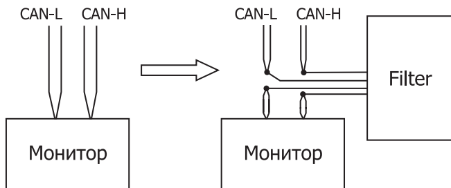
Рис. 3. Схема разрыва двойной шины CAN.
