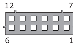
Рис. 2. Нумерация контактов в разъеме, вид со стороны проводов
