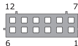
Рис. 2. Нумерация контактов в разъеме, вид со стороны проводов
