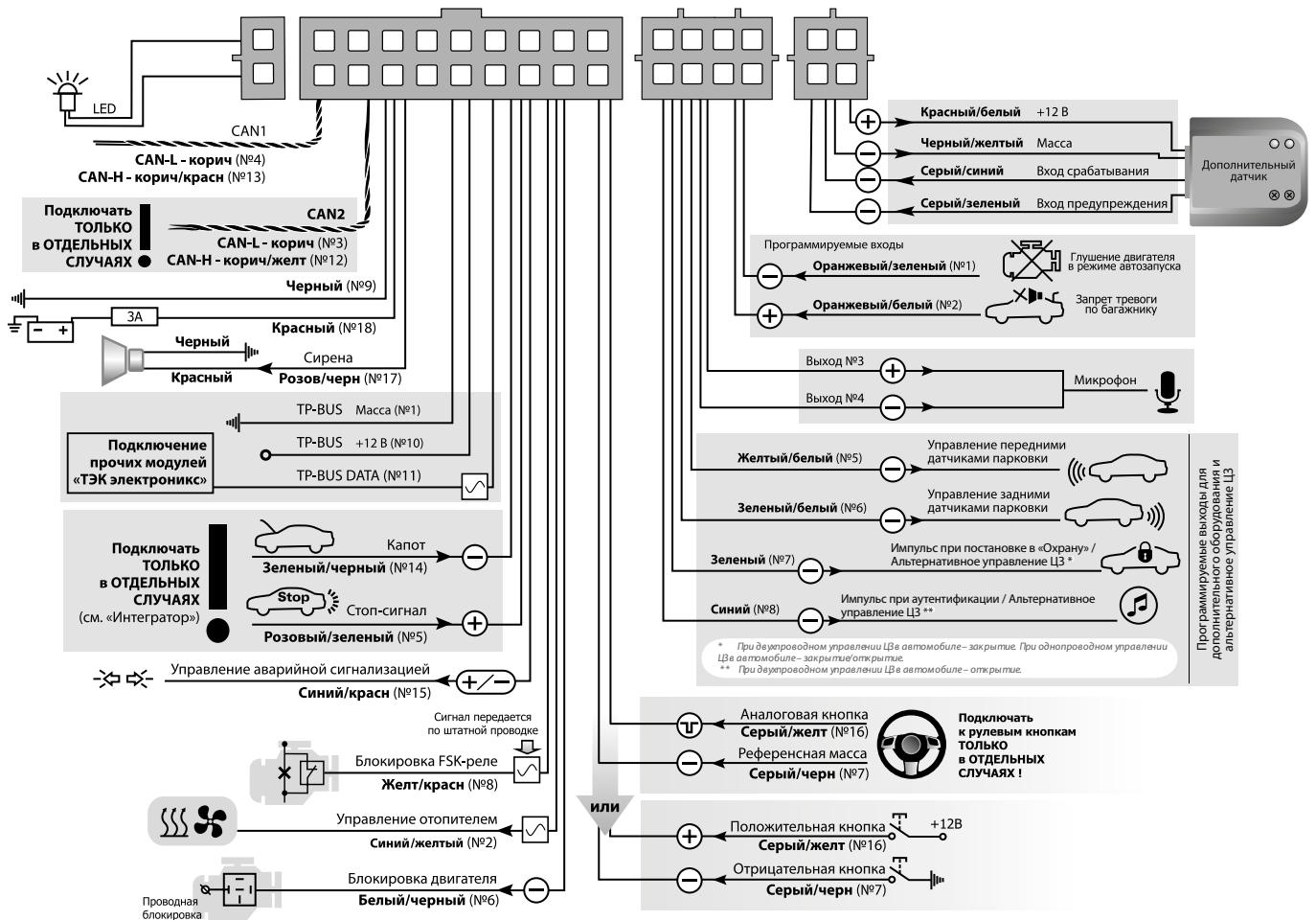
Схема подключения «Призрак»-820, 840
