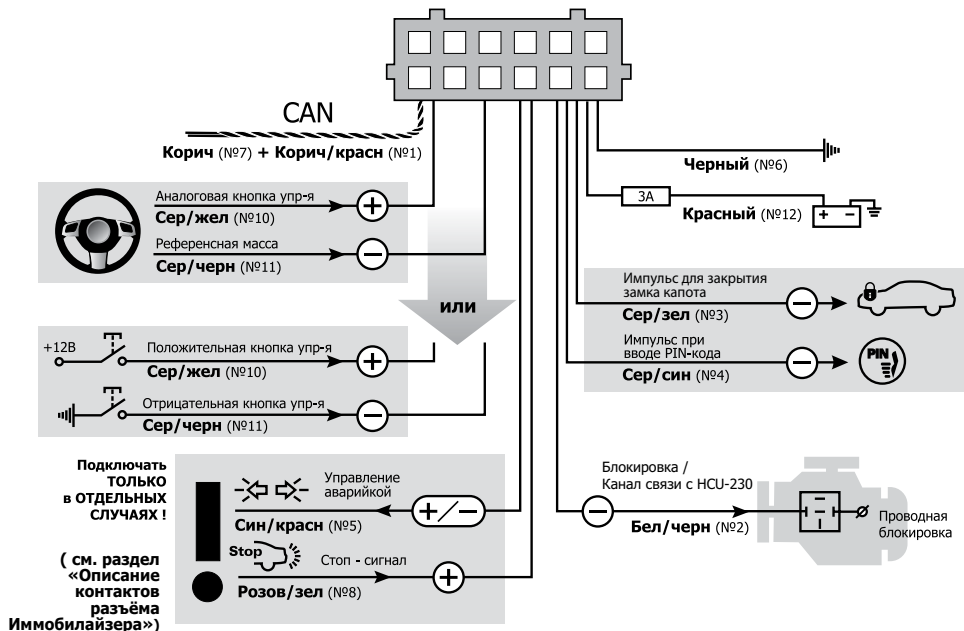
Схема подключения иммобилайзера «Призрак»-510 (заводские установки)
