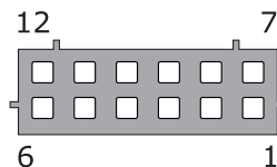
Рис. 3. Нумерация контактов в разъеме, вид со стороны проводов
