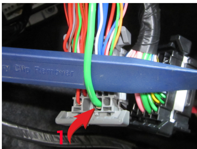
Подключение к цепям запуска двигателя 1 – Зажигание 2 (зеленый провод).
