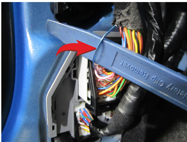
Место подключения (синий/черный провод, контакт N°41)
