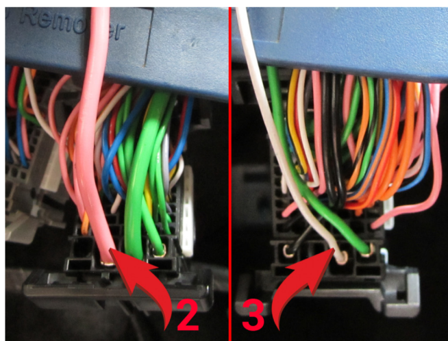
Подключение к цепям запуска двигателя 2 – Зажигание (розовый провод); 3 – Стартер (белый провод).
