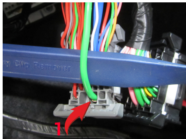
Рис.5 Подключение к силовым цепям 1 - Зажигание 2 (зеленый провод)
