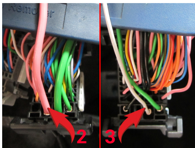
Рис.6 Подключение к силовым цепям 2 - Зажигание (розовый провод) 3 - Стартер (белый провод)
