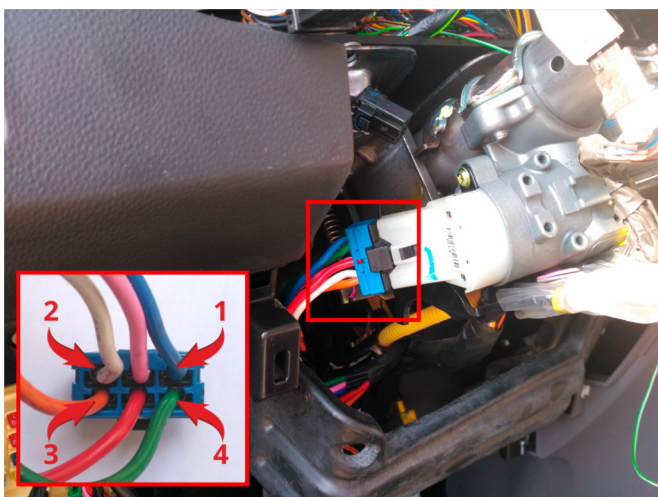
Подключение к силовым цепям запуска двигателя 1 – АСС (синий провод); 2 – Зажигание 1 (белый провод); 3 – Зажигание 2 (оранжевый провод); 4 – Стартер (зеленый провод).
