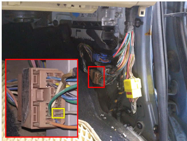
Место подключения (серый провод)
