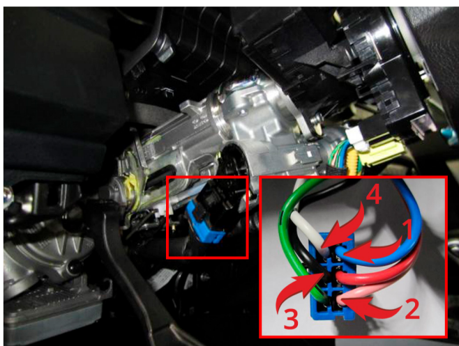
Подключение к силовым цепям запуска двигателя 1 – АСС (синий провод); 1 – Зажигание 1 (розовый провод); 2 – Зажигание 2 (черный провод); 3 – Стартер (белый провод).
