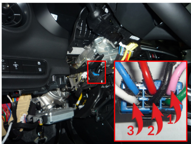
Подключение к силовым цепям замка зажигания 1 - Зажигание 1 (розовый провод); 2 - Зажигание 2 (черный провод); 3 - Стартер (белый провод).
