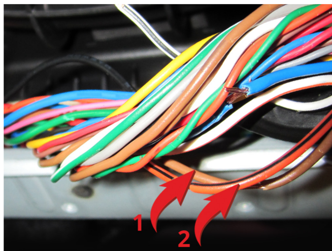
Подключение к силовым цепям запуска двигателя 1 - Зажигание 1 (коричневый провод); 2 - Зажигание 2 (оранжевый/фиолетовый).
