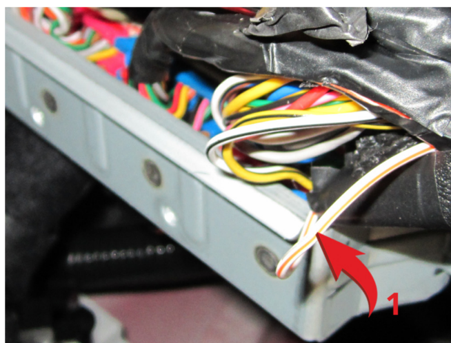
Подключение к силовым цепям запуска двигателя 1 - Стартер (белый/оранжевый провод)
