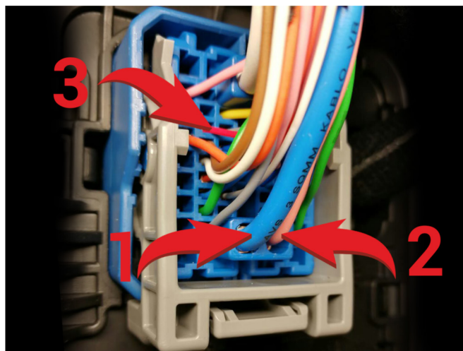
Подключение к цепям запуска двигателя 1 - Зажигание 1 (синий провод); 2 - Зажигание 2 (розовый провод); 3 - Стартер (красный провод).
