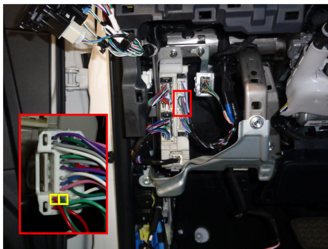
Место подключения
