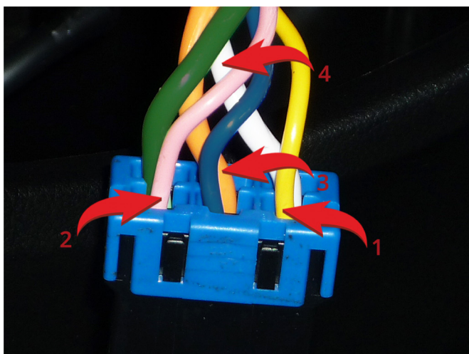
Подключение к силовым цепям запуска двигателя 1 – АСС (желтый провод); 2 – Зажигание 1 (розовый провод); 3 – Зажигание 2 (оранжевый провод); 4 – Стартер (белый провод).
