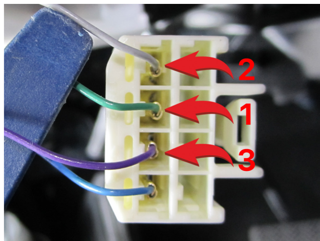
Подключение к цепям замка зажигания 1 - АСС (зеленый провод); 2 - Зажигание 1 (серый провод); 3 - Стартер (фиолетовый провод).
