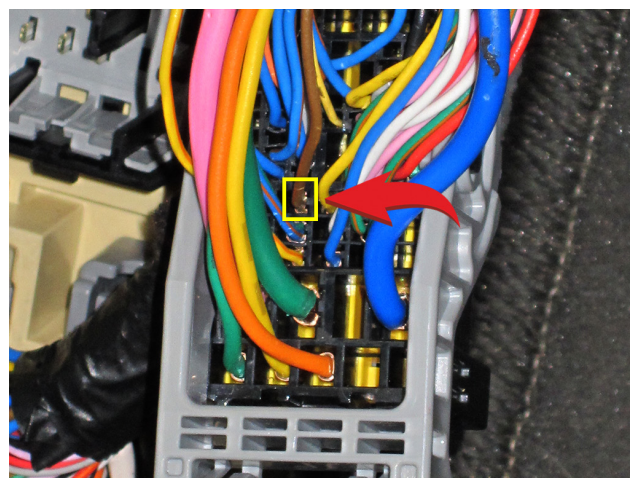
Рис.3 Шина данных (коричневый/оранжевый провод)
