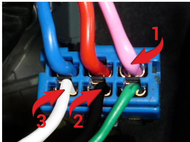
Рис.6 Подключение к силовым цепям запуска двигателя 1 – Зажигание 1 (розовый); 2 – Зажигание 2 (черный); 3 – Стартер (белый).
