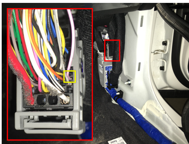
Шина данных (розовый провод, контакт №54)
