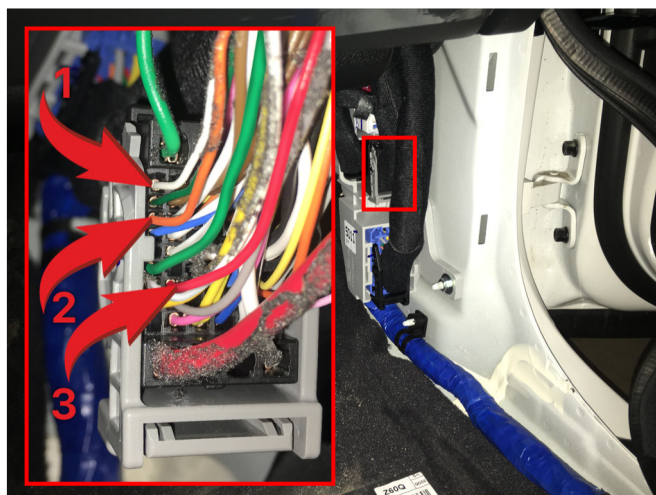
Подключение к силовым цепям замка зажигания 1 - Зажигание 1 (серый провод); 2 - Зажигание 2 (оранжевый провод); 3 - Стартер (красный провод).
